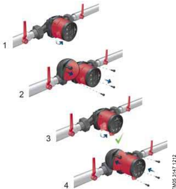
Fig. 5 Modification de la position du coffret de commande
