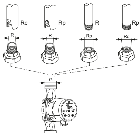
Fig. 43 Filetages G et filetages R
