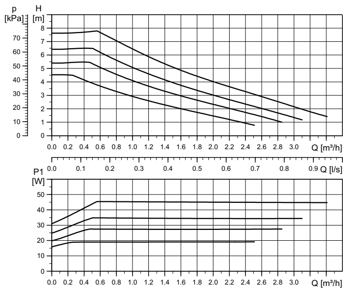
Fig. 51 Courbe de performance
