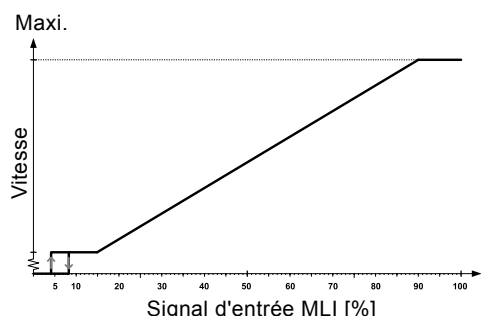
Fig. 48 Entrée MLI profil C
