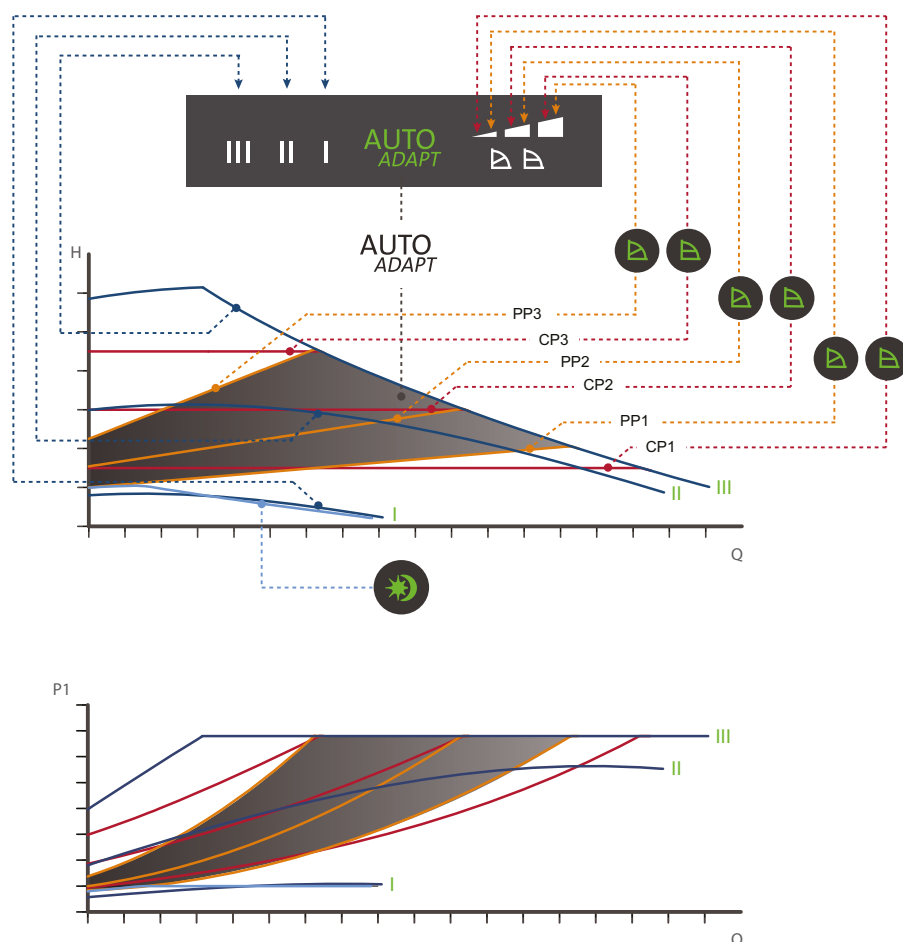
Fig. 36 Courbes de performance par rapport au réglage du circulateur
