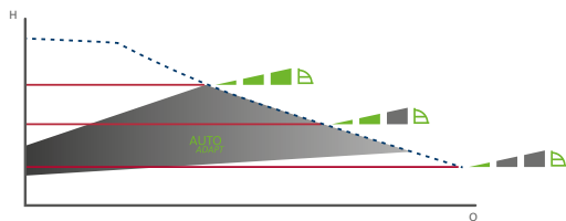
Fig. 25 Sélection du réglage du circulateur en fonction du type d'installation
