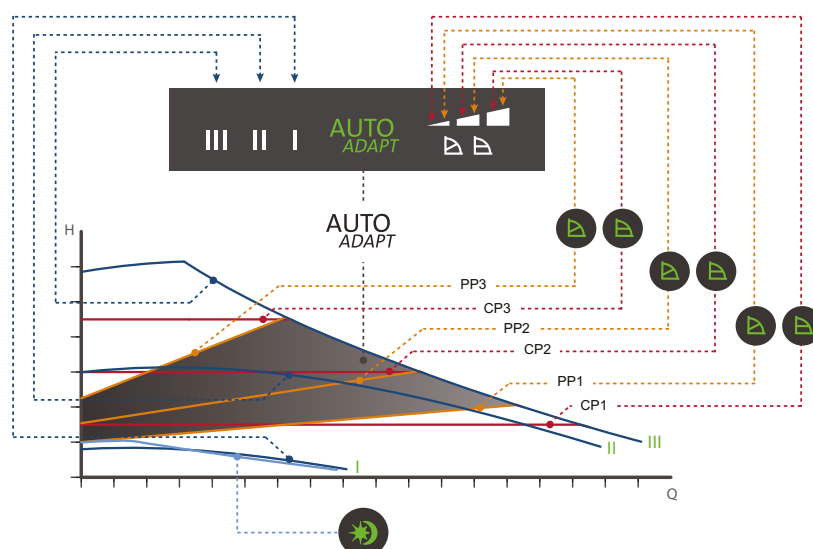
Fig. 29 Réglage du circulateur en fonction de ses performances
