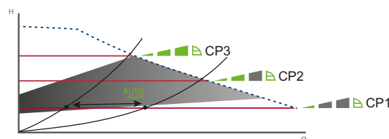
Fig. 24 3 courbes à pression constante et réglages
