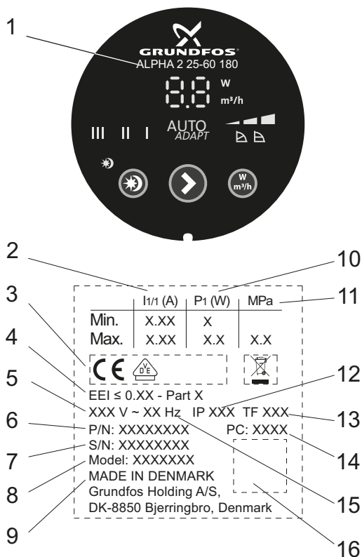
Fig. 18 Plaque signalétique
