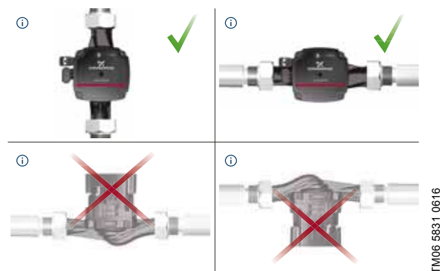
Fig. 7 Position du coffret de commande de l'ALPHA SOLAR
